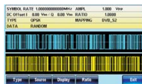
PSK
