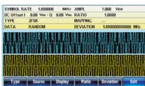
FSK
