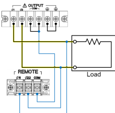
輸出與遙測連接示意圖
