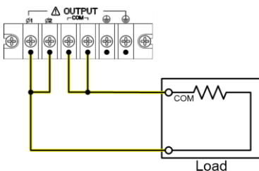
並聯輸出連接示意圖
